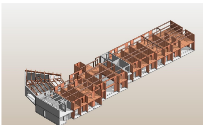
構造モデル(一部RC耐火構造にて別棟とし、準耐火不要とした)
