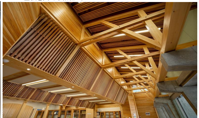
▼屋根を支える軸組トラス
